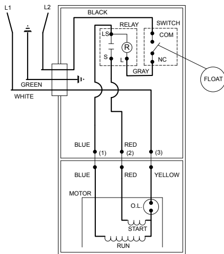
WIRING DIAGRAM FOR MODELS "M267-A", "M267-B", "M267-C", "M267-D", "D267-A", "D267-B", "D267-C", "D267-D" 4/79 (PI) thru 8/86 (US)
